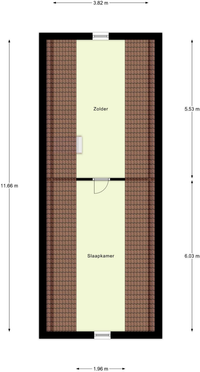
2e Verdieping/Zolder
