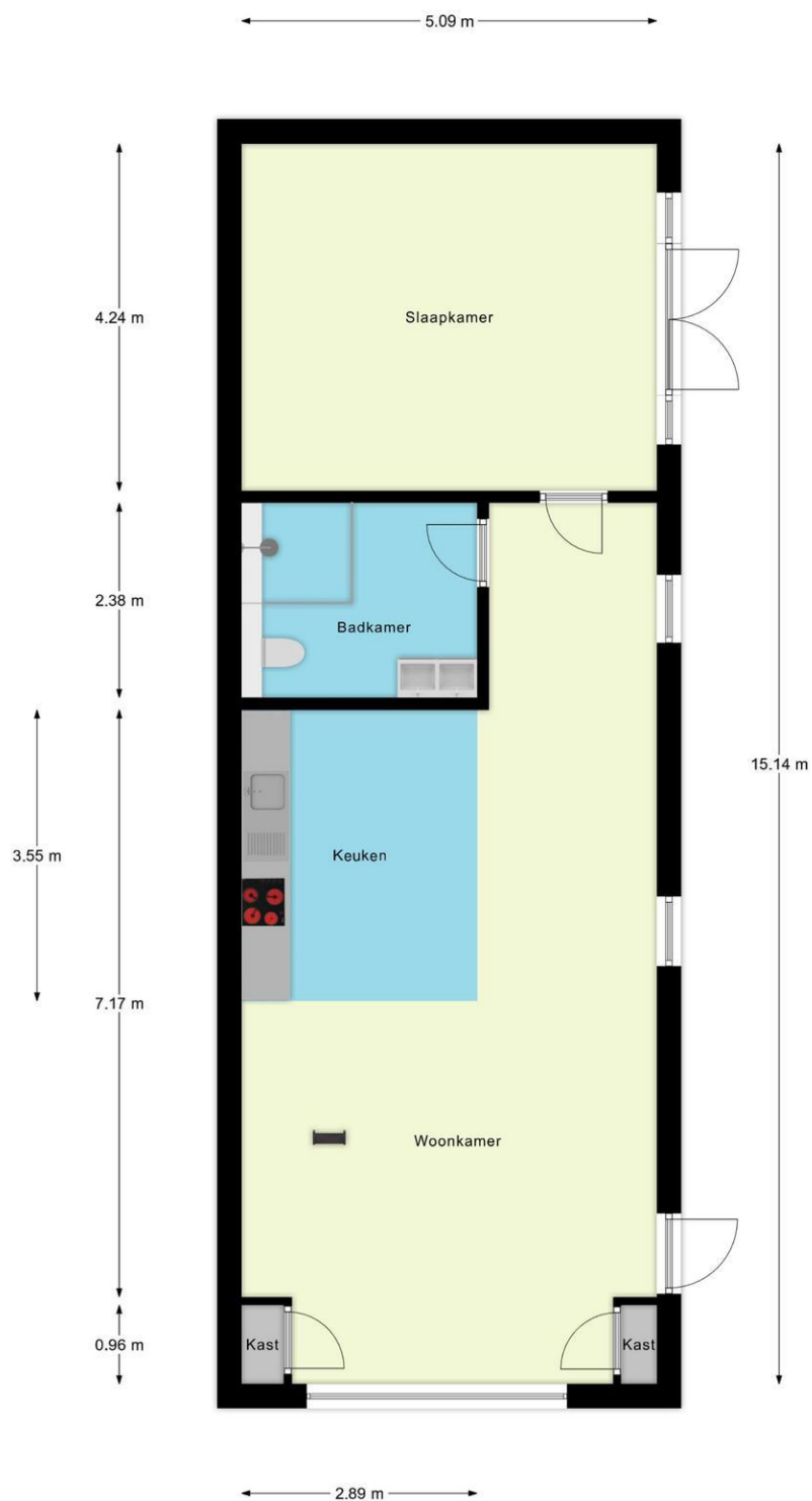
Garage Begane Grond/Aanleunwoning
