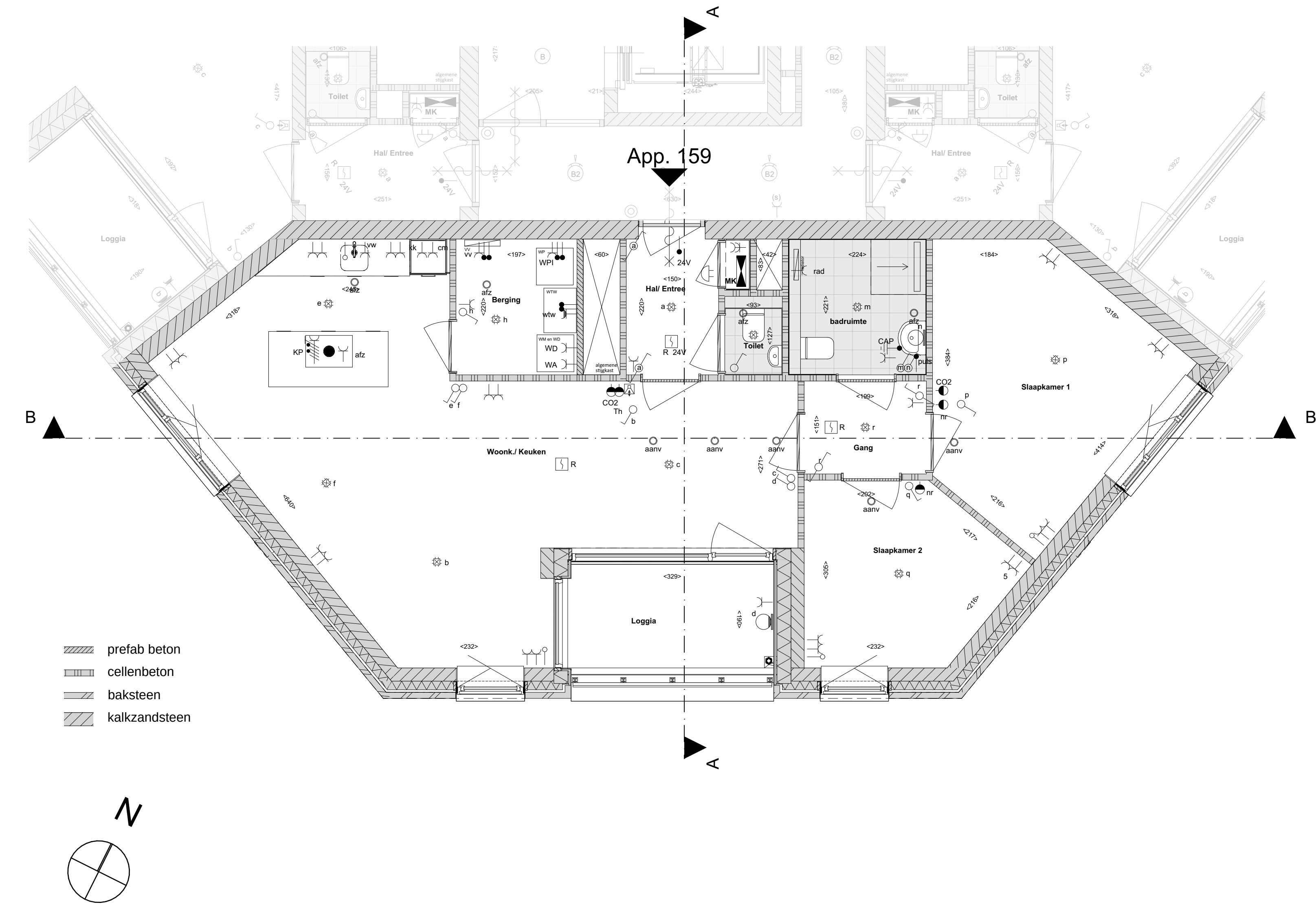
01 eerste verdieping | 1:50
