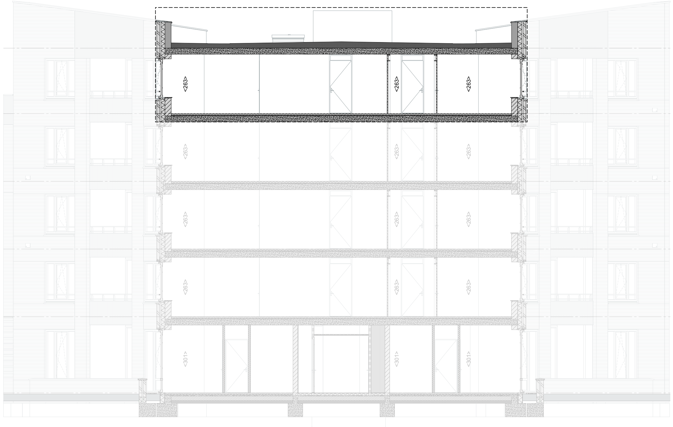
Doorsnede BB | 1:100
