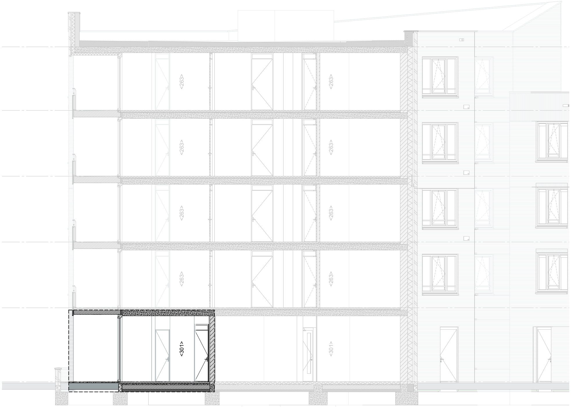
Doorsnede BB | 1:100
