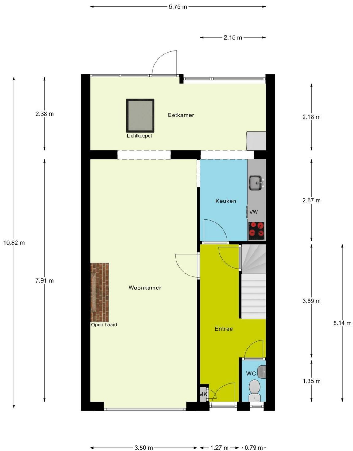
Begane Grond
