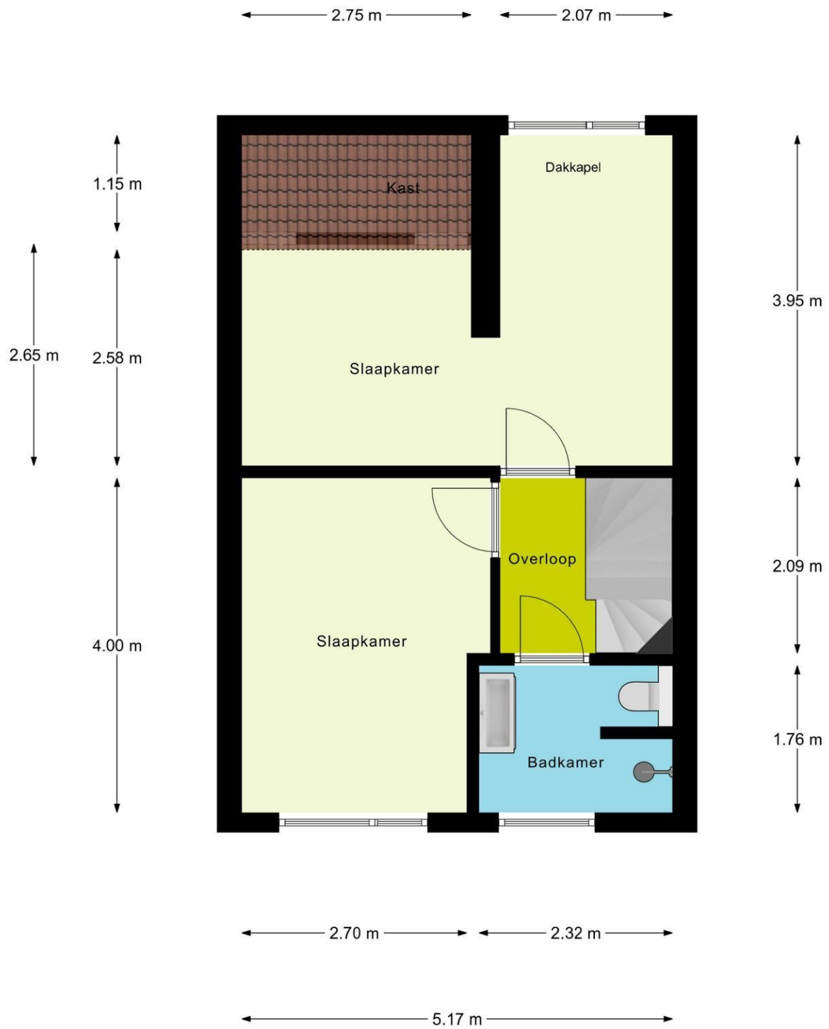
1e Verdieping
