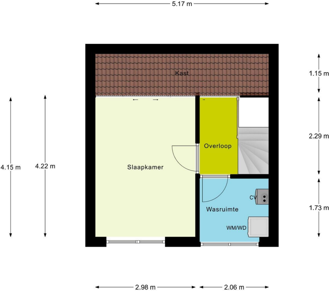
2e Verdieping
