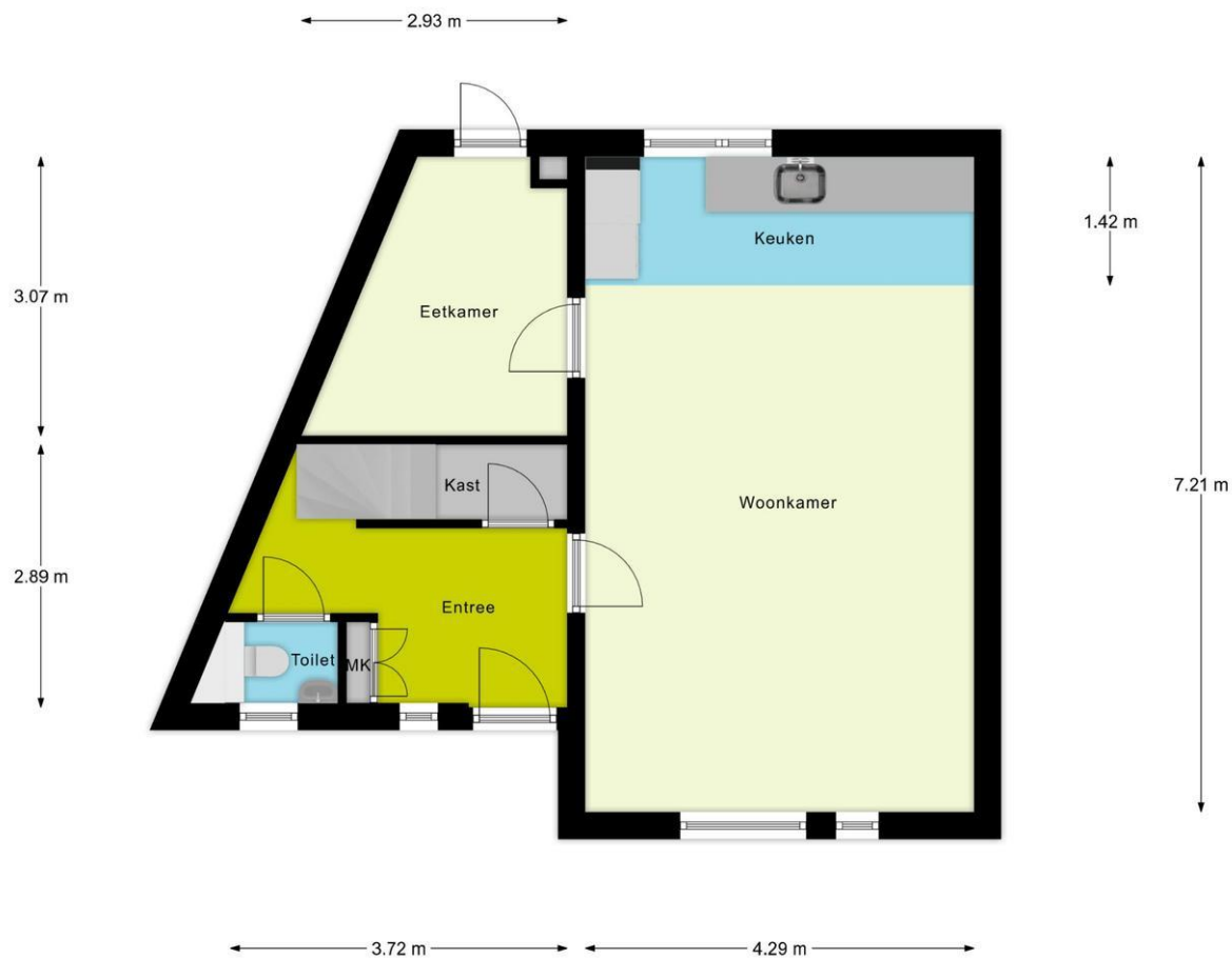
Begane Grond
