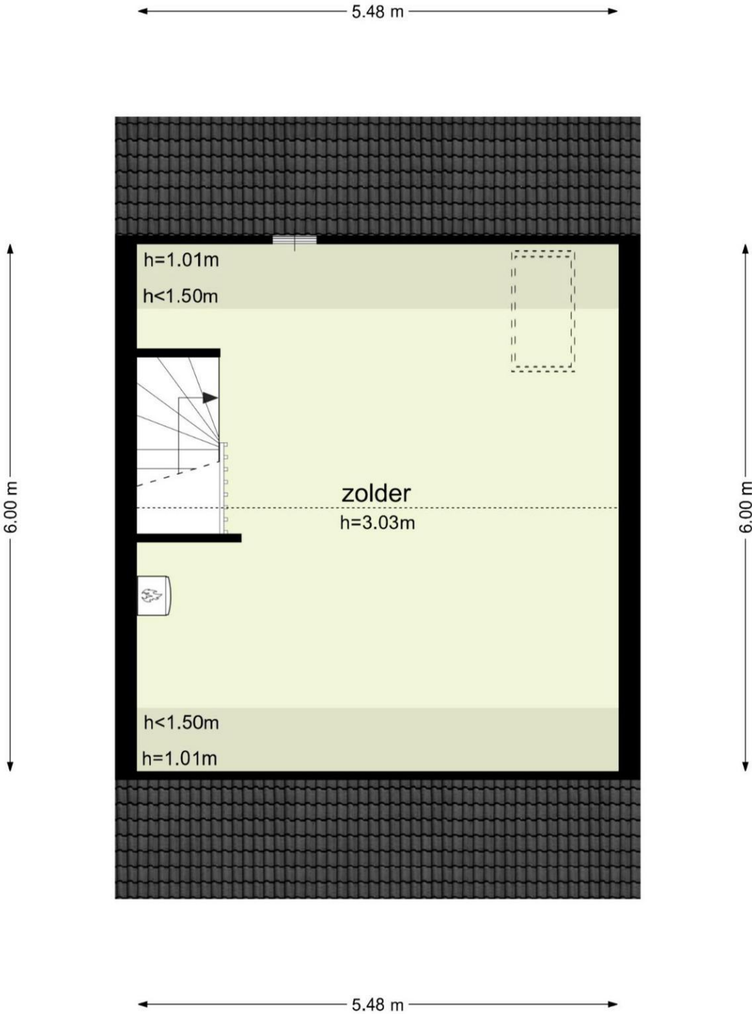
Tweede Verdieping
