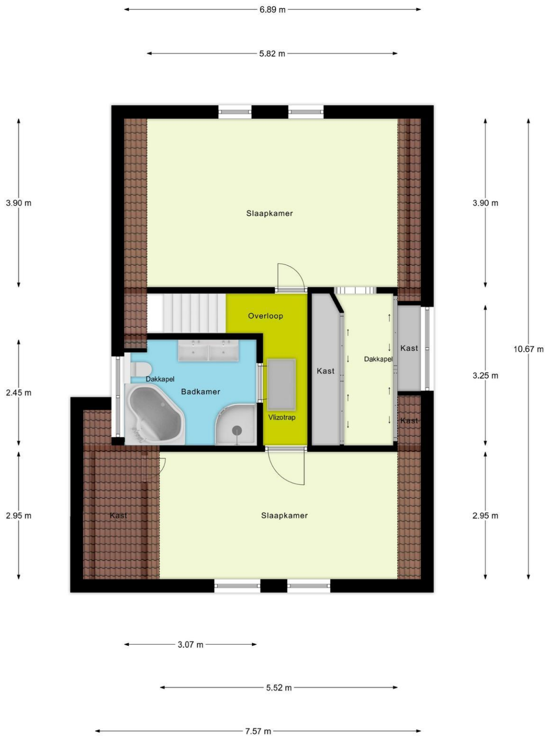
1e Verdieping
