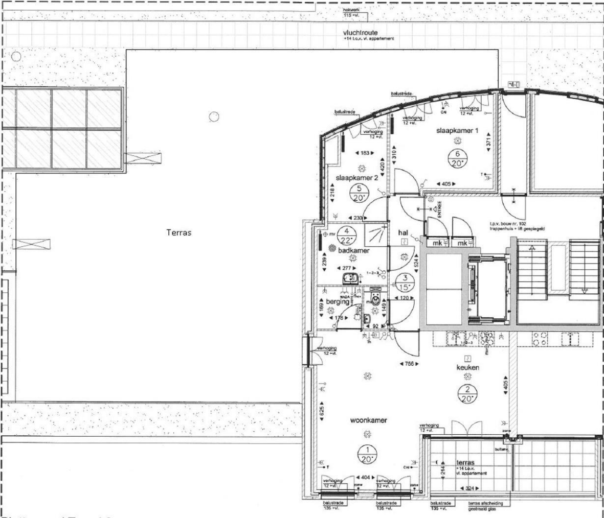
Plattegrond Type L3
