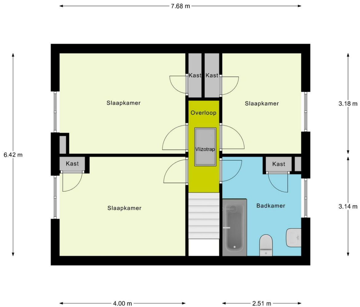
1e Verdieping
